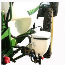
PREMEZCLADOR 40L CON LAVAENVASES Y SISTEMA ACERCAMIENTO USUARIO. (DE SERIE)
