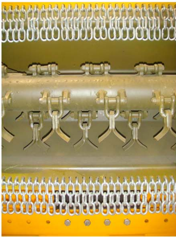
Rotor cuchillas o cuchillas con grillete
